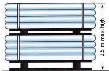
Frame packing of PE pipes
